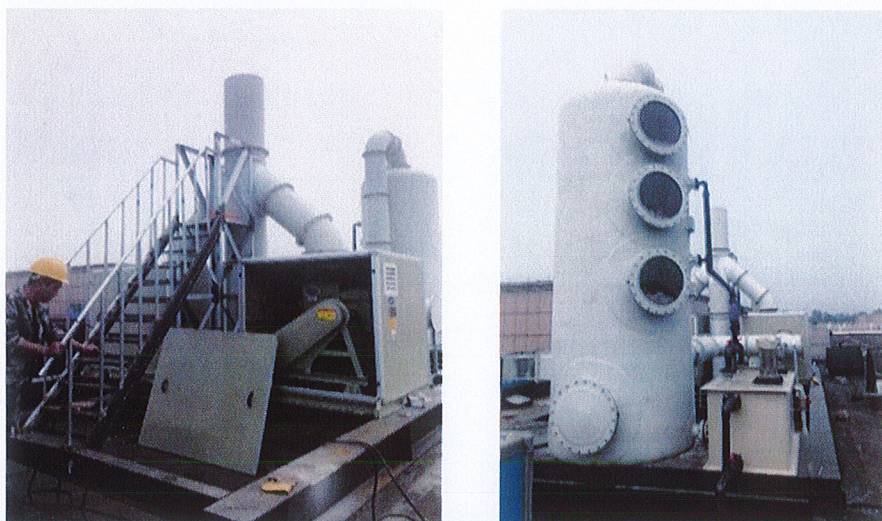
固体车间水喷淋废气治理设施
